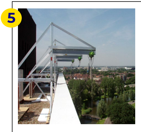
Overhang Optional
